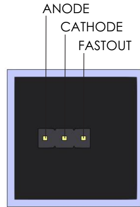
SCALE 4:1
